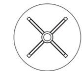
AD-989B(X脚) φ900・H690(t.12)(ガラス) H710(t.35)(木天板)
