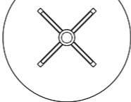
AD-989B(X脚) φ1200・H690(t.12)(ガラス) H710(t.35)(木天板)
