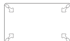
AD-152(150) W1500×D900×H700(t 35)
